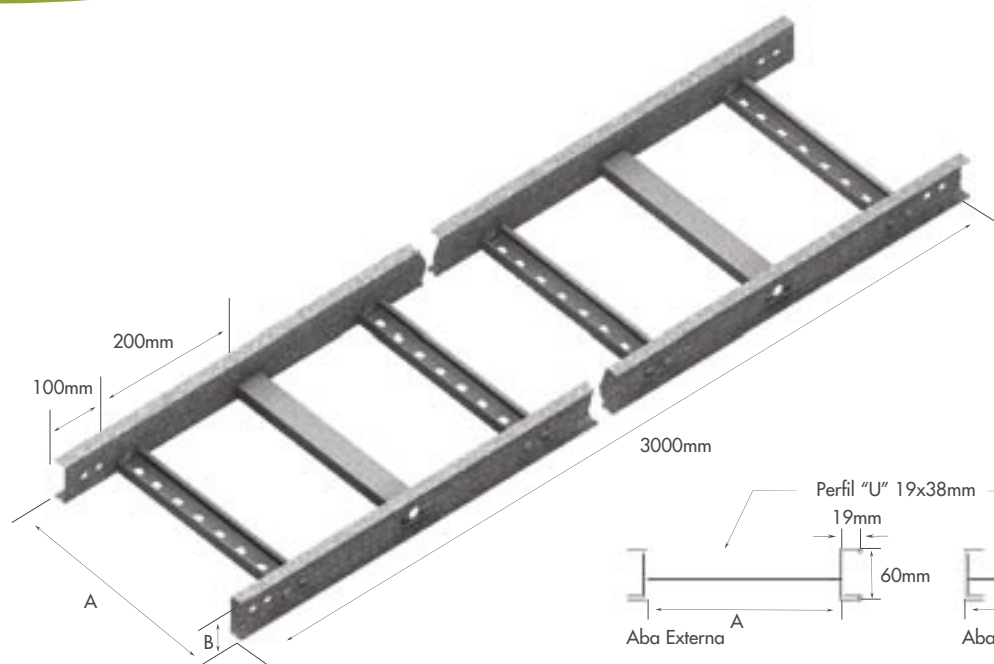
Leito para Cabo Tipo Leve Ref. CKL 600
