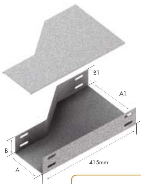
Redução à Esquerda Ref. CKE 538
