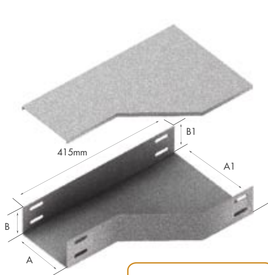
Redução à Direita Ref. CKE 537
