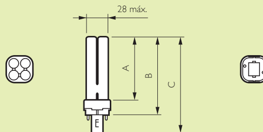
Diagramas de dimensões em mm
